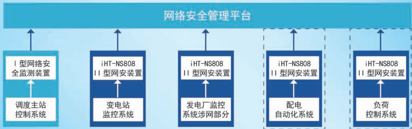
网络安全监视架构图
