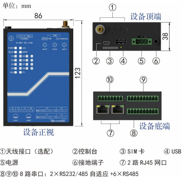
图 2-3 iHT-C24S 接线说明
