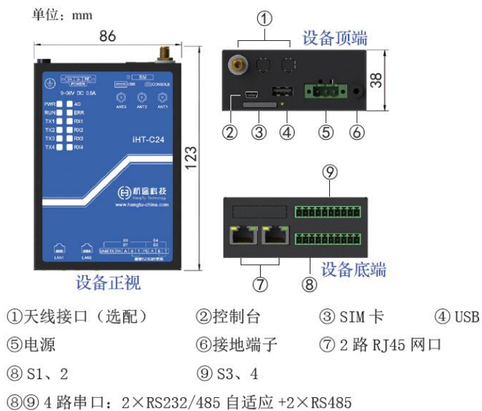
图 2-2 iHT-C24 接线说明
