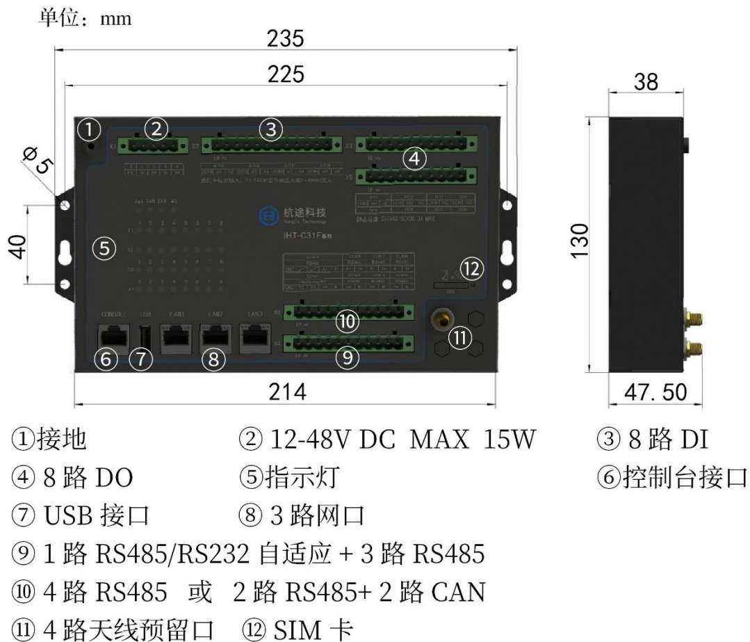
图 2-1 iHT-C31F 尺寸及接口说明图
