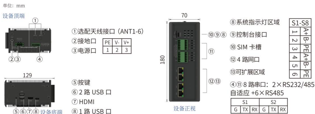
图 2-1 iHT-C61 接口示意图
