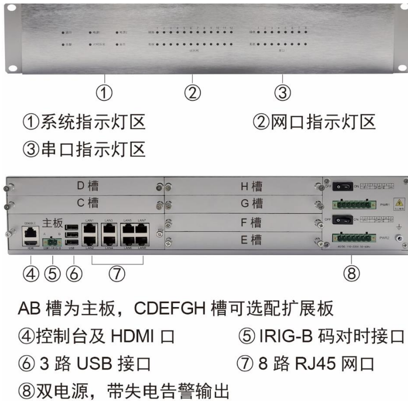
图 2-1 接口示意图
