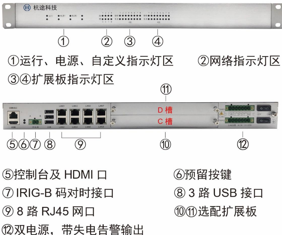
图 2-1 接口示意图
