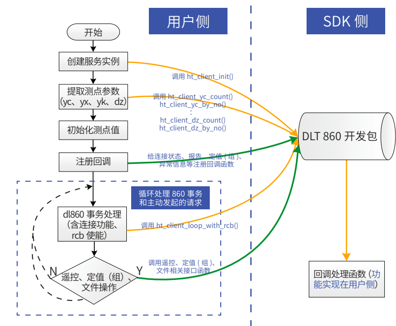
CMS 客户端接口调用流程图
