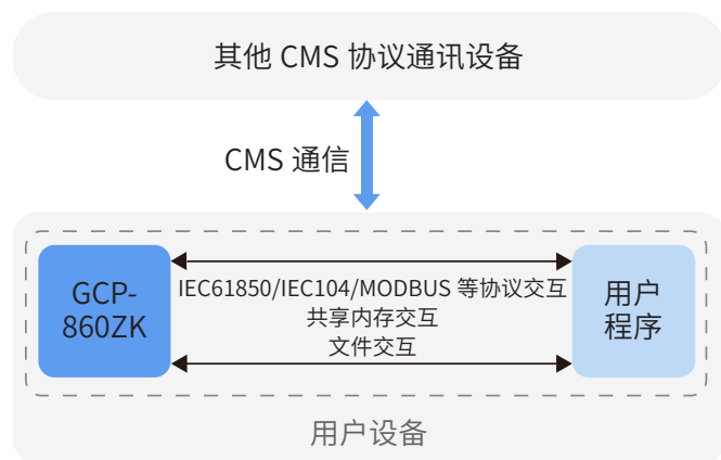
信息交互方案拓扑
