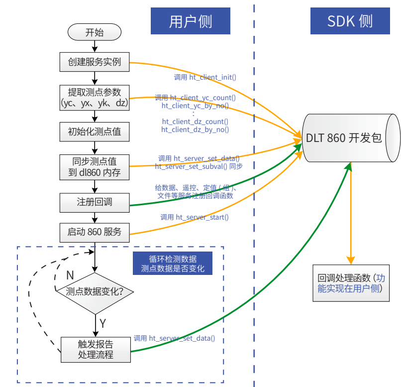
CMS 服务端接口调用流程图
